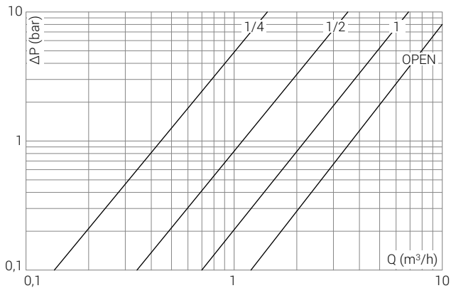
0318 0310 Valvole a squadra Angled radiator valves
